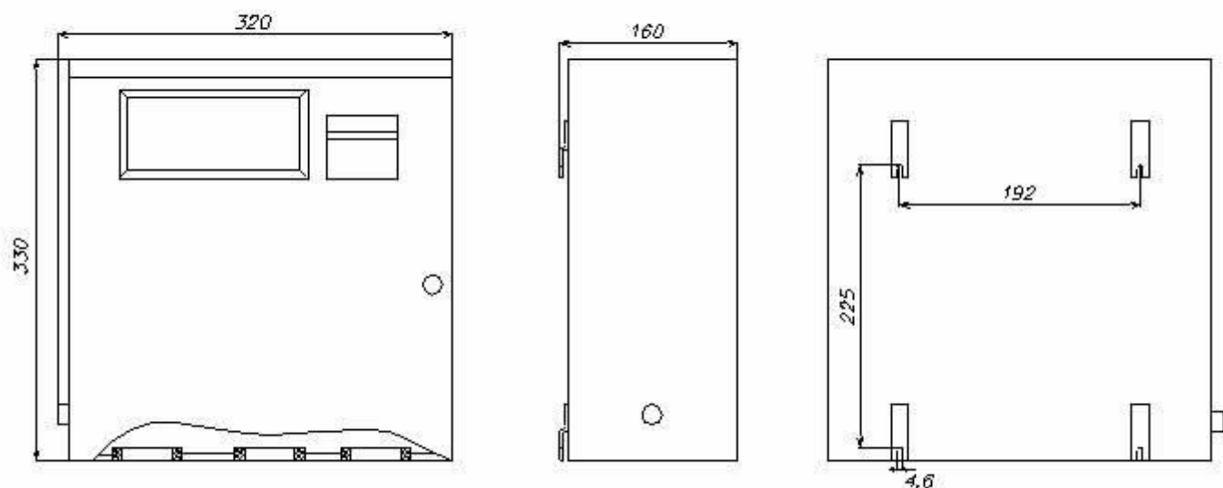
Габаритные и присоединительные размеры на станции управления СУЗ-10, СУЗ-25, СУЗ-40
